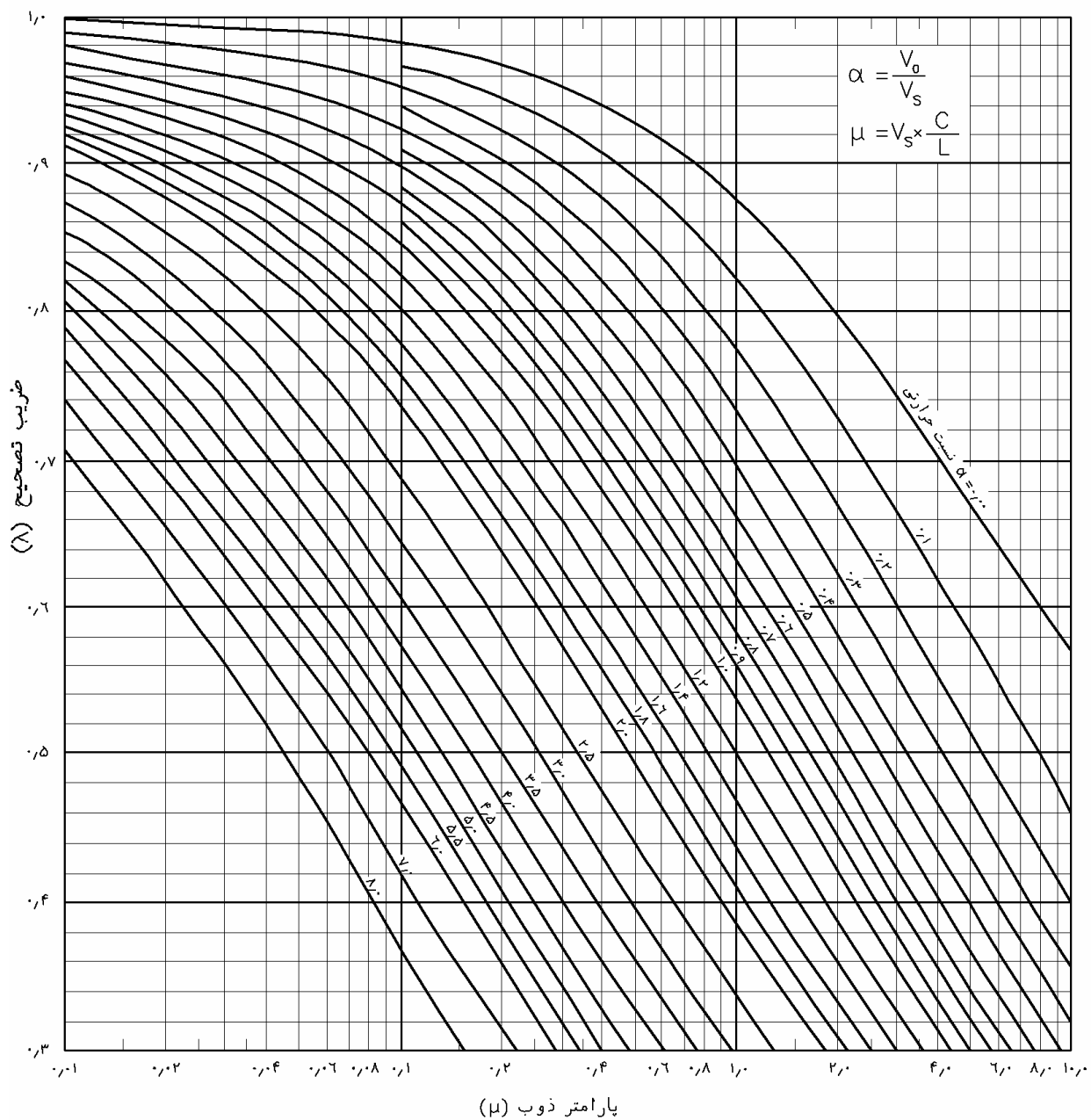
شکل پ-۲-۴- تعیین ضریب تصحیح λ در رابطه اصلاح شده برگرن 18
